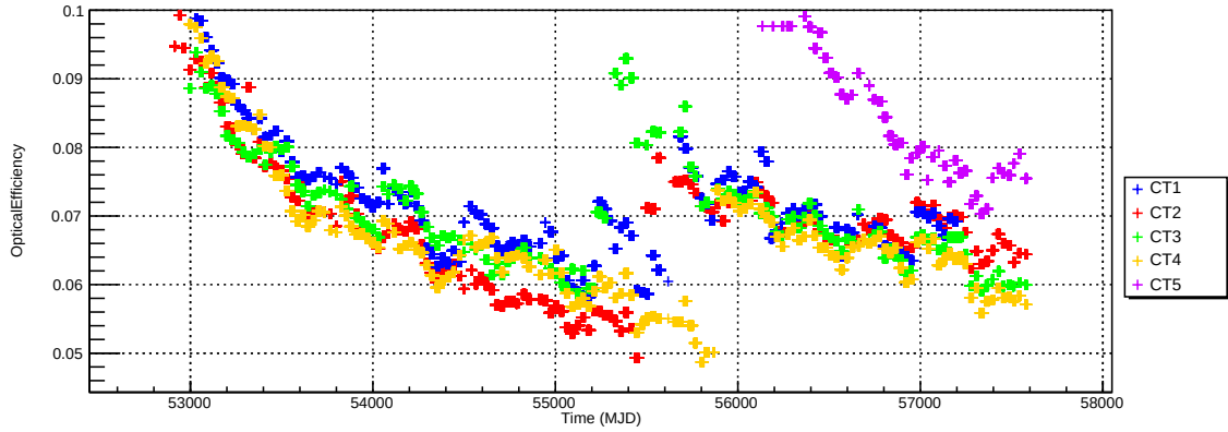
FIGURE 2.13 – Evolution de l'efficacité optique au cours du temps. La ré-aluminisation à partir de l'année 2011 a permis une augmentation significative de leur valeur.
