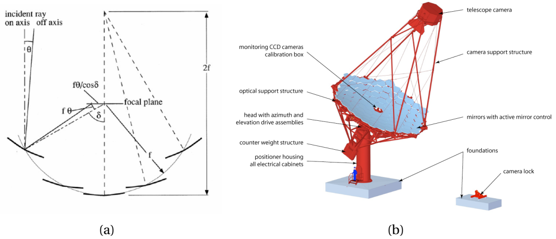
FIGURE 2.9 – (a) : Schéma de la configuration en Davies-Cotton [26], (b) : Le design du futur télescope MST de CTA aura également une configuration en Davies-Cotton [10].
