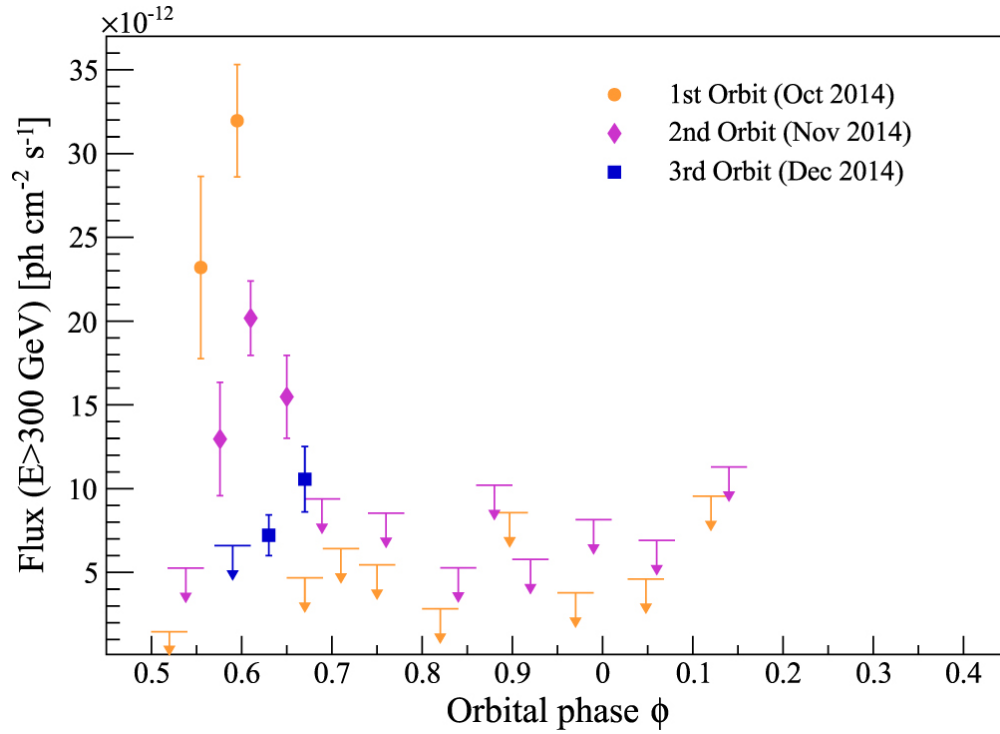
FIGURE 5.16 – Courbe de lumière de LS I +61 303 pendant la campagne d’observation de 2014 en fonction de la phase orbitale. Le graphe est représenté sur une période mais en prenant comme phase de départ 0.45. Les observations de VERITAS ont commencé autour de la phase de \phi = 0.5 pour chaque orbite. Les données pour la première orbite (octobre 2014) sont montrées avec des cercles orange, tandis que la deuxième orbite (novembre 2014) est représentée par des losanges violets, et la troisième (décembre 2014) par des carrés bleus. Les limites supérieures du flux avec un niveau de confiance de 99% (en utilisant l’approche de Rolke et al. [1]) sont montrées par des flèches [20].
