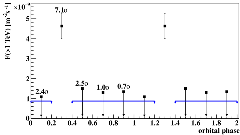
FIGURE 5.7 – Courbe de lumière rayonnée repliée sur la phase dans le domaine du TeV. La phase orbitale \Phi = 0.0 est définie au maximum de l'émission Fermi-LAT à \text{MJD} 57410.25 . Pour une meilleure lisibilité, deux orbites sont affichées. Le flux est calculé pour des intervalles de phase identique et une exposition similaire. Les barres d'erreur représentent 1 \sigma d'incertitude statistique. Les valeurs indiquées aux points de données indiquent la signification statistique de l'excès pour chaque de phase. Les lignes bleues désignent la limite supérieure (au niveau de confiance de 95%) sur le flux dans la région en dehors du pic (phase orbitale de 0.4 à 0.2) [50].
