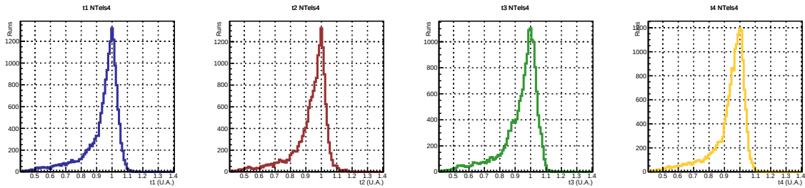
FIGURE 3.5 – Distribution du coefficient de transparence t_i pour une configuration H.E.S.S. I à 4 télescopes. Les courbes représentées correspondent en partant de la gauche vers la droite respectivement à CT1, CT2, CT3 et CT4. Des valeurs supérieures à 1 des coefficients de transparence traduisent une qualité exceptionnelle au moment de l'observation de l'atmosphère namibienne.
