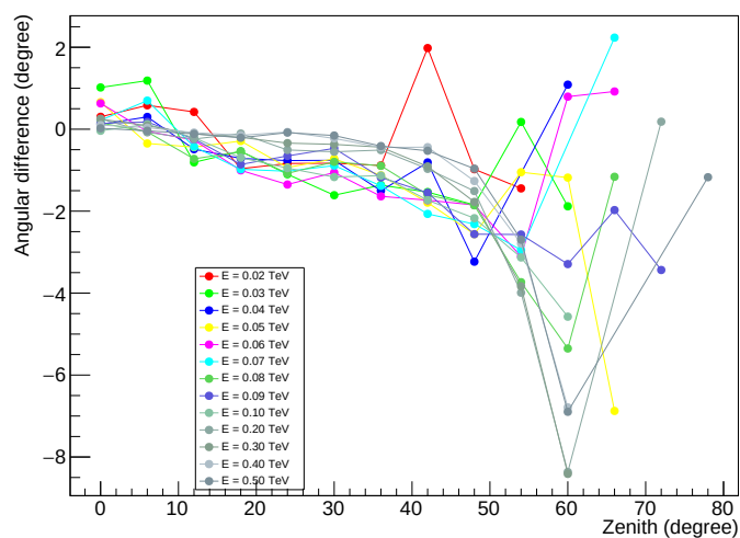
FIGURE B.6 – Influence de l'angle zénithal pour des gerbes en provenance de l'Ouest. L'angle d'impact est 0^\circ .
