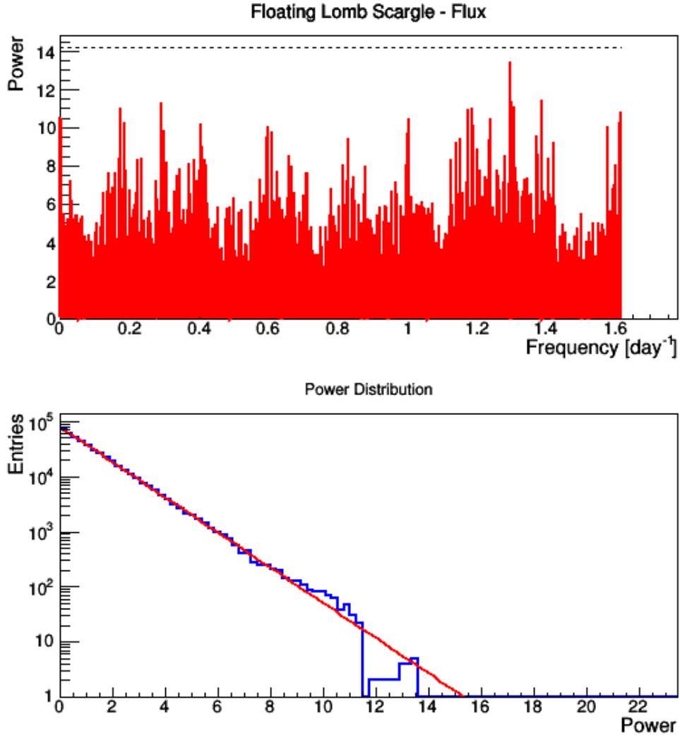
FIGURE 7.8 – Spectre de Fourier d'un signal où l'on a soustrait le signal modélisé du système binaire LS 5039 et distribution de z(\omega) par rapport au fond. La soustraction du signal permet de montrer que l'on obtient un spectre de Fourier aléatoire avec aucune valeur significative de la fonction normalisée z(\omega) . La distribution de z(\omega) est également ajustée par une fonction exponentielle f(x) = e^{(p_0 + p_1 \cdot x)} (en rouge). Les valeurs obtenues expérimentalement sont p_0 = 11.228 \pm 0.003 et p_1 = -0.734 \pm 0.001 .
