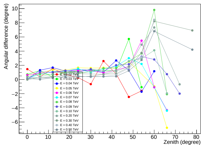
FIGURE B.7 – Influence de l'angle zénithal pour des gerbes en provenance de l'Ouest. L'angle d'impact est 0^\circ .
