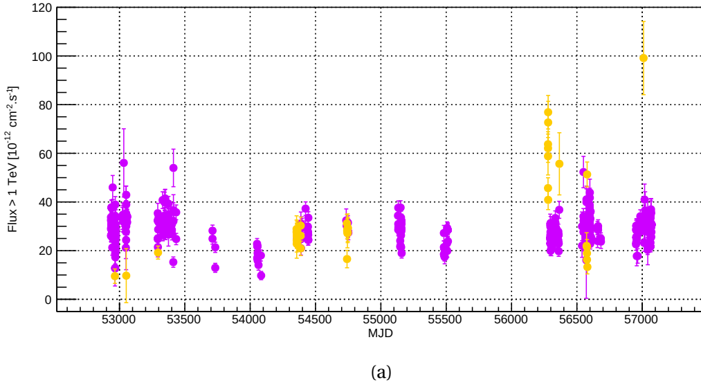
FIGURE 3.22 – Courbe de lumière de la nébuleuse du Crabe après correction par le coefficient de transparence. Les observations pour lesquelles TC < 0.70 sont toujours représentées en orange, mettant en évidence une surestimation de cette modification du flux pour certaines données.
