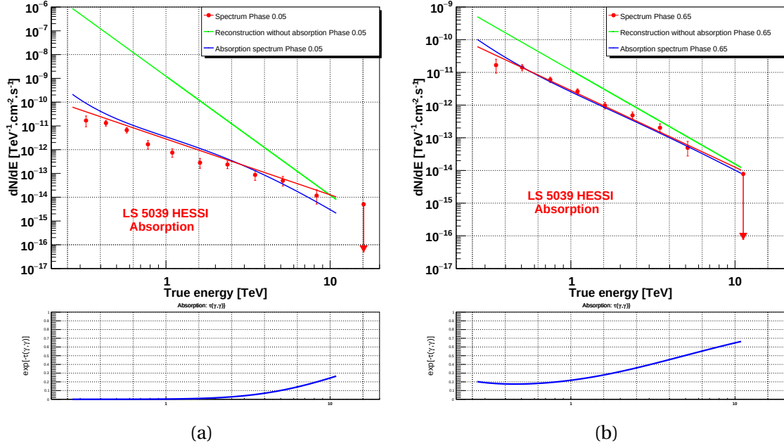
FIGURE 7.18 – Spectres d'absorption et de désorption de LS 5039. Sur les deux courbes, nous avons représenté le spectre avec une loi de puissance simple (en rouge), le spectre avec la loi de puissance avec le phénomène d'absorption (en bleu) et le spectre désorbé (en vert). La courbe \exp(-\tau_{\gamma\gamma}) est représentée à chaque fois en-dessous du spectre. L'angle d'inclinaison est supposé à chaque fois de 20^\circ . (a) : spectre de la phase 0.00 - 0.10 et (b) : spectre de la phase 0.60 - 0.70
