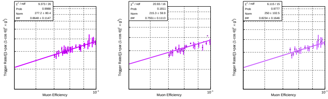
(b) Variation du taux de déclenchement en fonction l'efficacité optique \mu La fonction f(\mu) = \frac{R}{g^\beta \cdot [1 + \lambda(1 - \cos \theta)^2]} = k_5 \cdot \mu^\alpha est ajustée par un modèle en loi de puissance.
