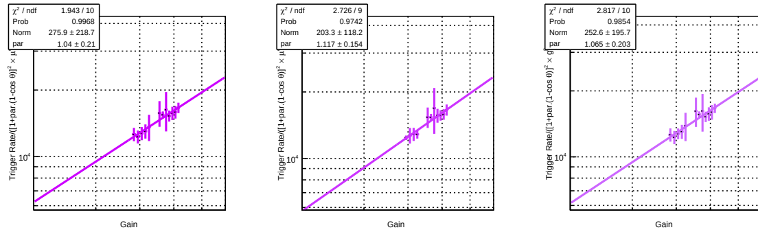
(c) Variation du taux de déclenchement en fonction du gain g . La fonction f(g) = \frac{R}{\mu^\alpha \cdot [1 + \lambda(1 - \cos \theta)^2]} = k_6 \cdot \mu^\alpha est ajustée par un modèle en loi de puissance
