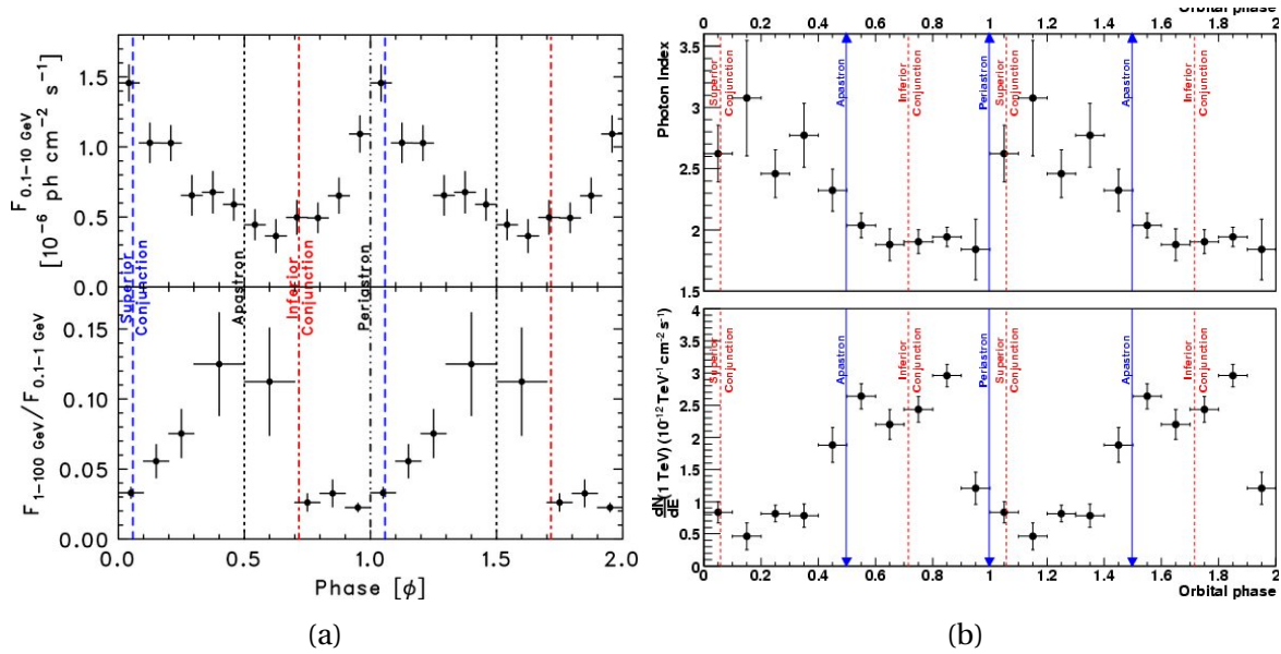
FIGURE 5.4 – Étude du flux obtenu par les expériences Fermi-LAT (a) et H.E.S.S. (b) respectivement pour le système LS 5039. (a) : courbe de lumière en fonction de la phase de l'objet compact, le flux est intégré sur 0.1 et 10 GeV. La courbe du bas indique le ratio entre la courbe de lumière sur le domaine 1 – 100 GeV et la courbe de lumière sur le domaine 0.1 – 1 GeV [2]. (b) : flux différentiel à 1 TeV et indice spectral en fonction de la position de l'objet compact, on observe une anticorrélation entre le flux et l'indice spectral. Sur le domaine II y a inversion du comportement de la source selon l'énergie considérée : le flux est minimal autour de la conjonction inférieure sur l'intervalle 0.1 – 10 GeV, mais il est maximal à 1 TeV [12].
