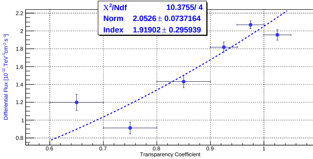
FIGURE A.9 – Influence de la transparence de l’atmosphère sur le flux différentiel mesuré de LS 5039 à 1 TeV.
