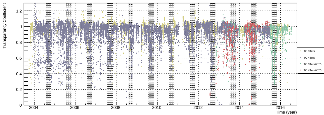
FIGURE 3.11 – Evolution temporelle du coefficient de transparence. Le coefficient de transparence est déterminé à partir des quatre configurations étudiées H.E.S.S. phase I à 4 télescopes en bleu, H.E.S.S. phase I à 3 télescopes en brun, H.E.S.S. phase II à 5 télescopes en rouge et H.E.S.S. phase II à 4 télescopes en cyan. On remarque une dégradation régulière de l'atmosphère pendant les mois d'août, septembre et octobre. Ces périodes sont représentées par des bandes grises sur le graphe.
