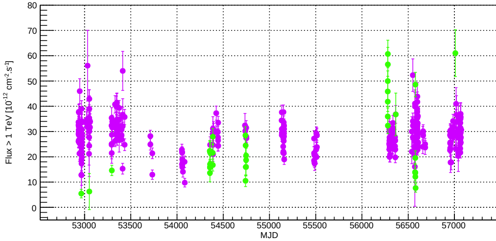
FIGURE 3.23 – Répartition des valeurs de la courbe de lumière avant et après correction par le coefficient de transparence. Les grandeurs dont TC < 0.70 sont représentées en vert, elles sont corrigées par une valeur fixe \Phi_{Cor} = \frac{\Phi}{0.70^{1.79}} évitant ainsi une surestimation de cette correction contrairement à la figure 3.22.
