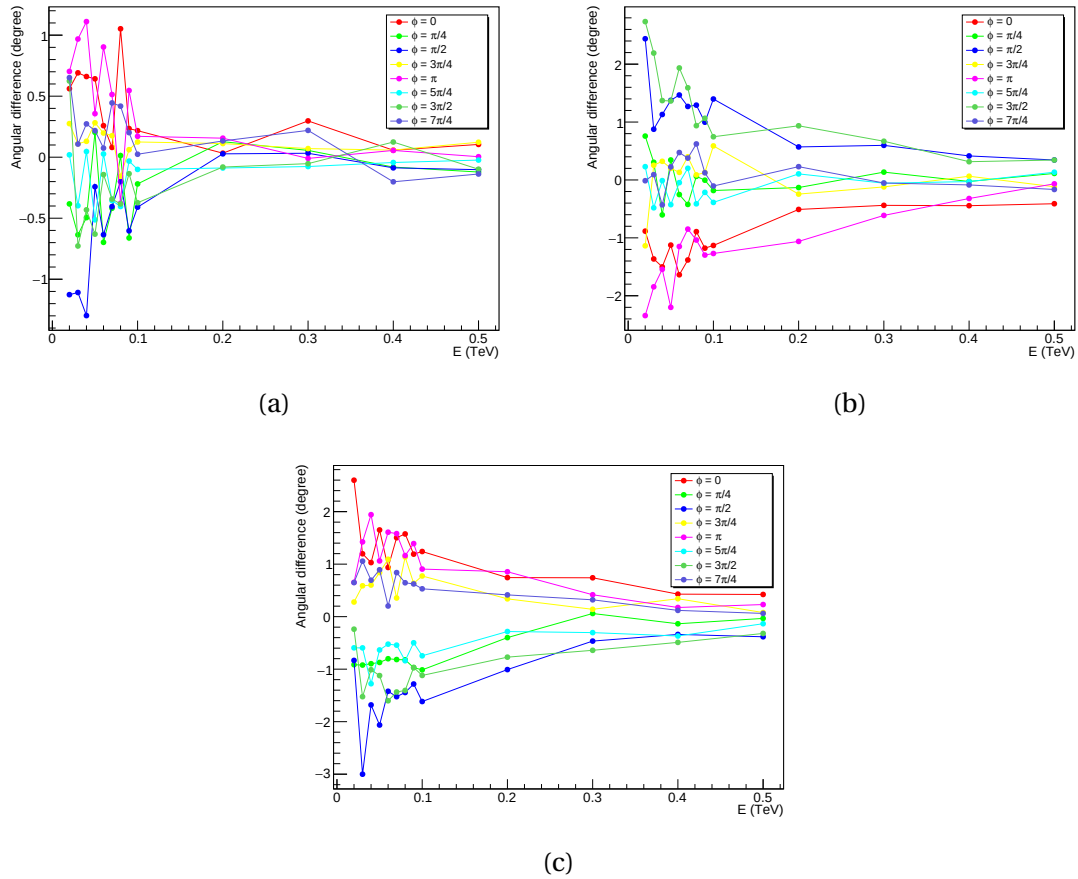
FIGURE B.1 – Influence de l'énergie du photon sur la rotation de la gerbe selon différents angles d'impact et directions azimuthales : (a) Nord, (b) Ouest et (c) Est. L'angle zénithal choisi est à chaque fois de 36^\circ .
