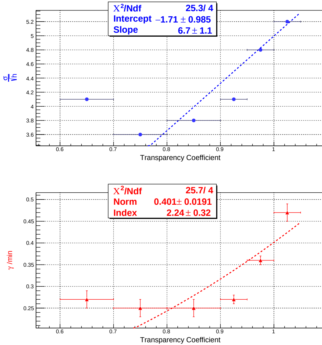
FIGURE 7.19 – Influence du coefficient de transparence sur la valeur de la signification du système binaire LS 5039 corrigée par le temps ( \frac{\sigma}{\sqrt{h}} ) et sur le nombre de photons \gamma détectés par minute (figure du bas). La courbe est ajustée selon une droite linéaire pour la figure du haut et une loi de puissance pour la figure du bas.
