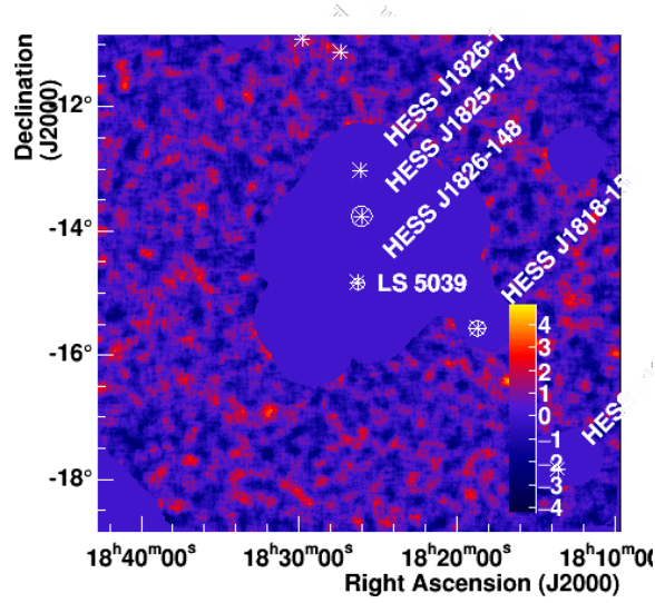
FIGURE 7.1 – Carte des régions d'exclusion de LS 5039 et signification du fond. Les zones à exclure de l'analyse sont représentées par des tachées violettes uniformes, elles occupent une aire importante sur la carte. Les autres régions (régions OFF) présentent une signification relativement faible assurant ainsi moins de systématiques sur la détermination du flux.
