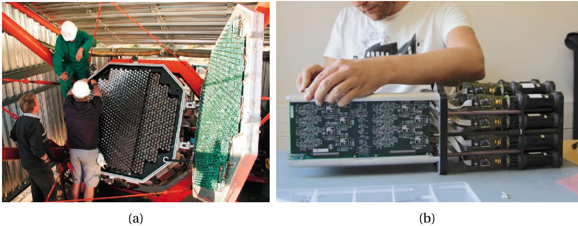
FIGURE 2.10 – (a) : Photo d'une des caméras de H.E.S.S. au moment de l'installation des cônes de Winston, (b) : Assemblage d'un module des nouvelles caméras de H.E.S.S. en Namibie, montrant de droite à gauche les photodétecteurs avec leurs bases et la carte de lecture, avec leurs puces NECTAr.
