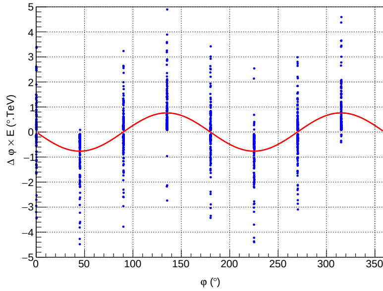
FIGURE 4.10 – Influence de l'angle d'impact sur la rotation de l'image dans la caméra. Pour certains angles d'impact, ce paramètre n'a aucun effet.
