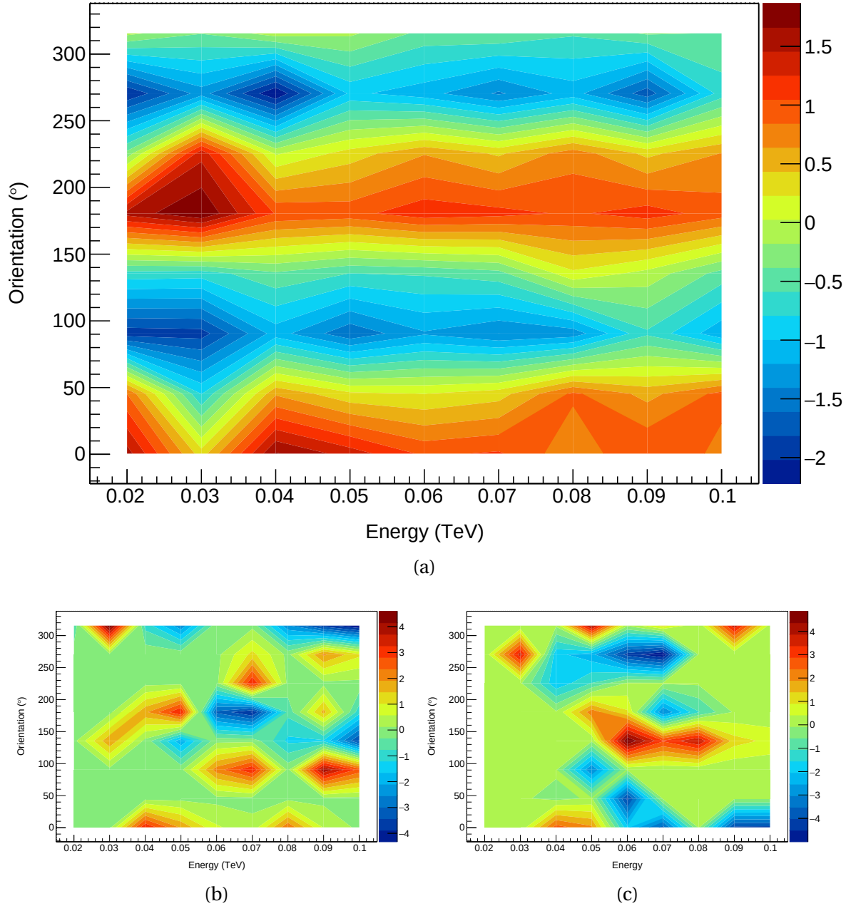
FIGURE 4.6 – Variation angulaire, de largeur et de longueur de l'ellipse en fonction de l'énergie du photon simulée pour un angle zénithal de 12^\circ provenant du Sud. Sur l'axe des abscisses est représenté l'énergie du photon, l'axe des ordonnées l'angle d'impact du photon et en couleur la variation du paramètre étudié. (a) : variation angulaire \Delta\phi , (b) : variation relative de la longueur \Delta L et (c) : variation relative de la largeur \Delta L .
