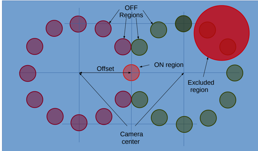
FIGURE 2.15 – Méthode de soustraction en utilisant la technique des régions OFF multiples. La caméra a pointé dans la zone de la source étudiée (ON region) à deux endroits différents (croix bleues). Les régions OFF (en vert et en violet) ont la même taille et se situent à la même distance du centre de la caméra que la région ON. On a représenté une région d'exclusion, ce qui a pour effet de supprimer deux régions OFF.
