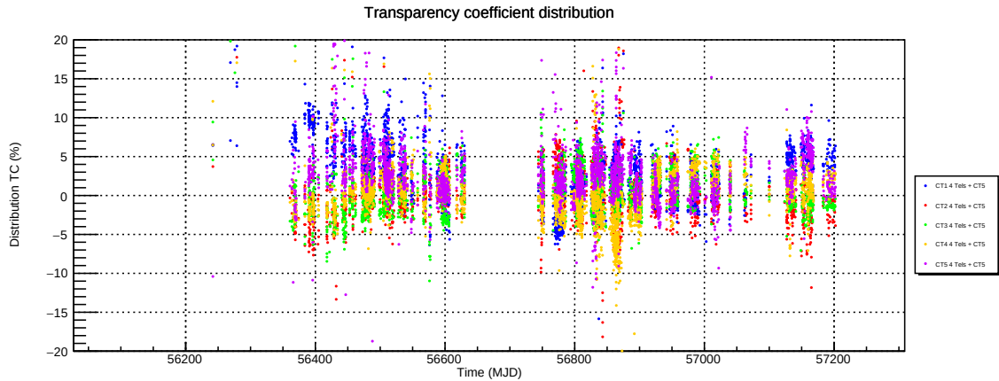
FIGURE 3.9 – Écart relatif du coefficient de transparence pour chaque télescope pour une configuration H.E.S.S. phase II à 5 télescopes. Cet écart relatif est représenté en bleu pour CT1, en rouge pour CT2, en vert pour CT3, en orange pour CT4 et en violet pour CT5.
