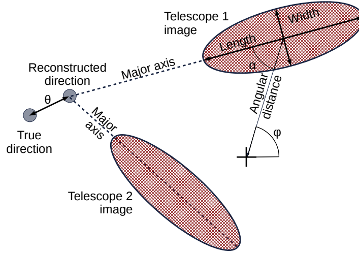
FIGURE 2.14 – Définition des paramètres de Hillas. L'intersection des axes principaux des ellipses à partir de plusieurs télescopes permet de reconstruire la direction de la source.
