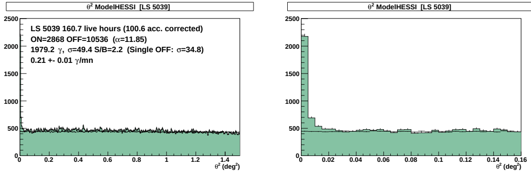
FIGURE 7.3 – Détermination du \theta^2 de la source pour une analyse H.E.S.S. phase I. Le graphe de droite montre un zoom au niveau de la source du même graphe.
