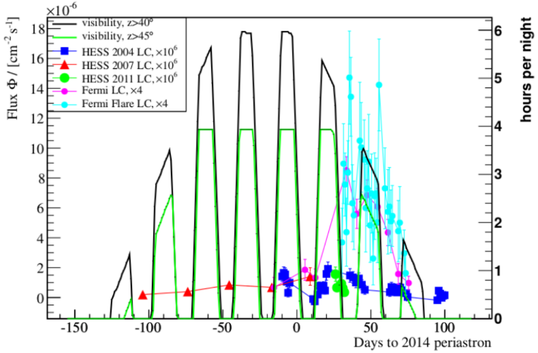
FIGURE 8.1 – Visibilité de PSR B1259–63 depuis le site de H.E.S.S. pendant la campagne d’observation de 2014 et comparaison des courbes de lumière des précédents passages et de l’éruption détecté par Fermi.
