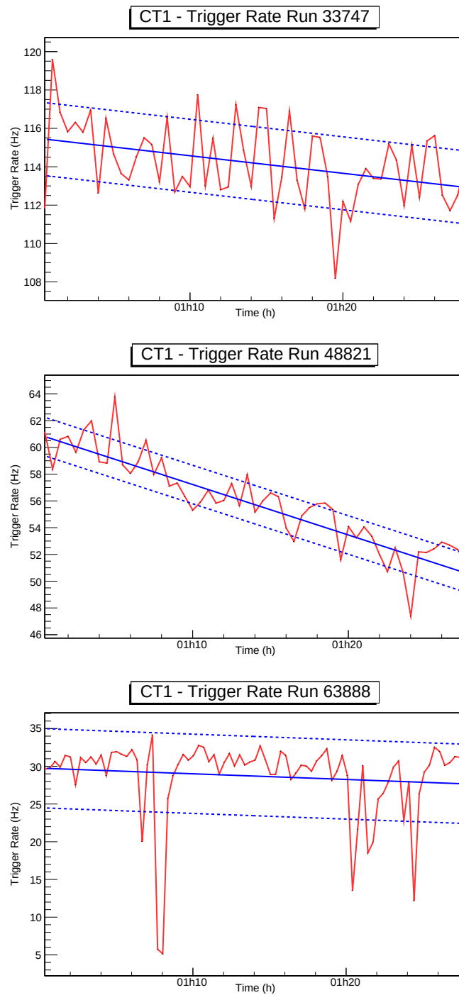
FIGURE 3.2 – Variation du taux de déclenchement du télescope 1 au cours de plusieurs observations (ligne continue en rouge) 33747, 48821 et 63888. La droite représentée en bleu représente une modélisation de cette variation du taux de déclenchement selon une régression linéaire. Les droites bleus en pointillés représentent une dispersion de 1\sigma autour de la droite modélisée (variable R_{\text{dispersion}} ).
