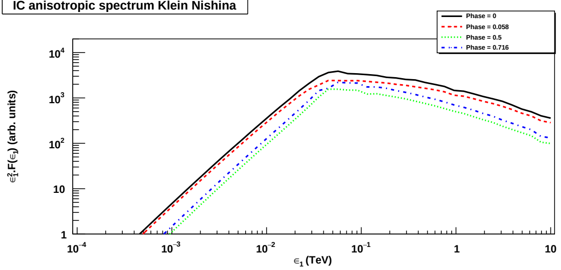
FIGURE 6.6 – Modélisation du spectre LS 5039 dans le cas d'une diffusion inverse Compton en régime de Klein-Nishina pour une inclinaison de 30^\circ et aux mêmes positions particulières de l'objet compact que pour la figure 6.5. Les échelles d'énergie sont différentes. Les fluctuations de la courbe correspondant à la conjonction supérieure correspondent à des incertitudes de la simulation.
