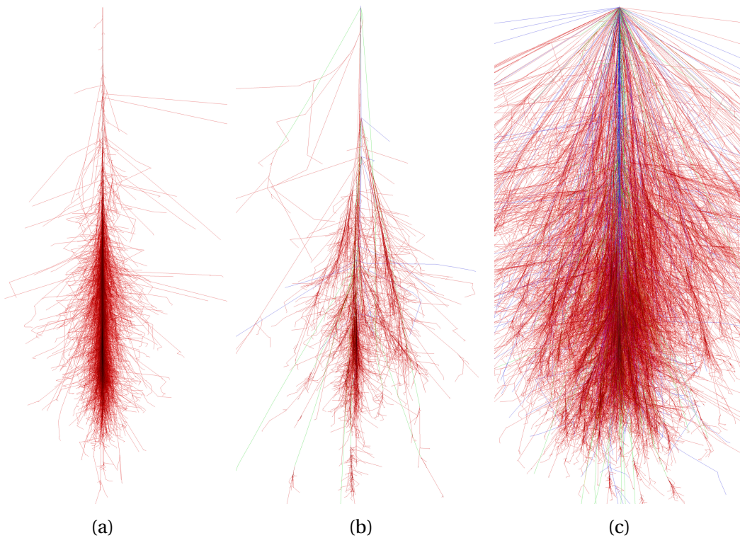
FIGURE 2.4 – Simulations de cascades atmosphériques engendrées par un photon à 100 GeV (a), un proton à 100 GeV (b) et un noyau de fer à 1 TeV (c) avec un angle zénithal nul. [13] [14]
