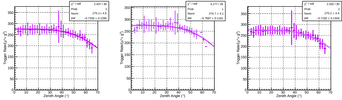
(a) Variation du taux de déclenchement en fonction l'angle zénithal \theta . La fonction f(\theta) = \frac{R}{g^\beta \cdot \mu^\alpha} = k_4 \cdot [1 + \lambda(1 - \cos \theta)^2] est ajustée selon un modèle parabolique.
