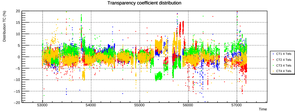
FIGURE 3.8 – Écart relatif du coefficient de transparence pour chaque télescope pour une configuration H.E.S.S. phase I à 4 télescopes. Cet écart relatif est représenté en bleu pour CT1 (moins visible à cause des autres points), en rouge pour CT2, en vert pour CT3 et en orange pour CT4. Pour certaines périodes, l'écart devient plus important notamment juste après la ré-aluminisation des télescopes.
