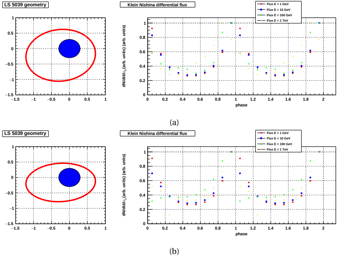
FIGURE 6.7 – Flux différentiel de phase simulé pour différentes énergies (1 GeV en rouge, 10 GeV en bleu, 100 GeV en vert et 1 TeV en jaune) selon la phase de l'objet compact pour le système binaire LS 5039 avec une orbite inclinée de 30^\circ (a) ou de 50^\circ (b) par rapport à l'observateur. Pour des inclinaisons plus élevées, le profil de la modulation change à des énergies plus élevées.
