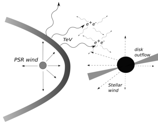
FIGURE 5.8 – Schéma montrant l'interaction entre un vent de pulsar et le vent ou le disque d'une étoile Be. Le processus synchrotron et le processus Inverse Compton par l'intermédiaire du choc avec le vent du pulsar produisent respectivement des rayons X et des rayons \gamma au TeV. Les rayons \gamma s'ils sont suffisamment énergétiques peuvent créer de nouvelles paires d'électrons et de positrons par le processus de création de paires de photons-photons, et ils peuvent générer ainsi une cascade de création de paires, dans la direction de l'étoile de compagnon [74].
