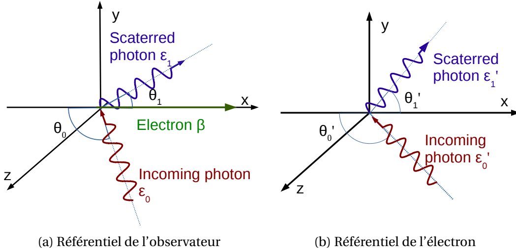
FIGURE 6.1 – Diffusion d'un photon dans le référentiel de l'observateur (a) et dans le référentiel de l'électron (b).
