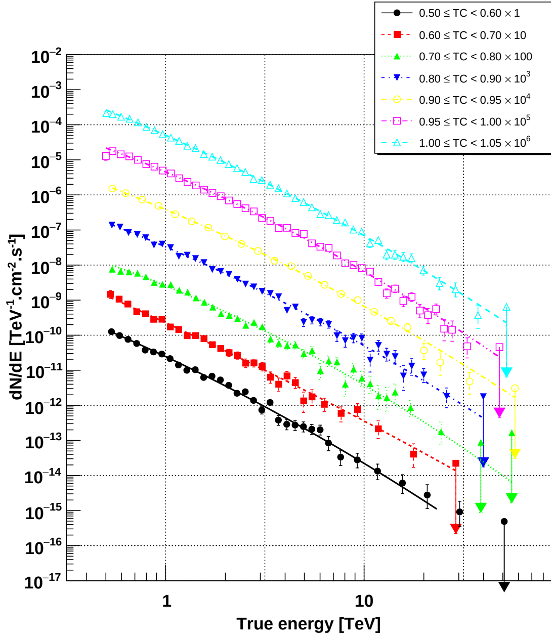
FIGURE 3.18 – Spectres de la Nébuleuse du Crabe en loi de puissance courbée pour différentes valeurs du coefficient de transparence. Les courbes ont été espacées d'un facteur dix pour plus de lisibilité du spectre.
