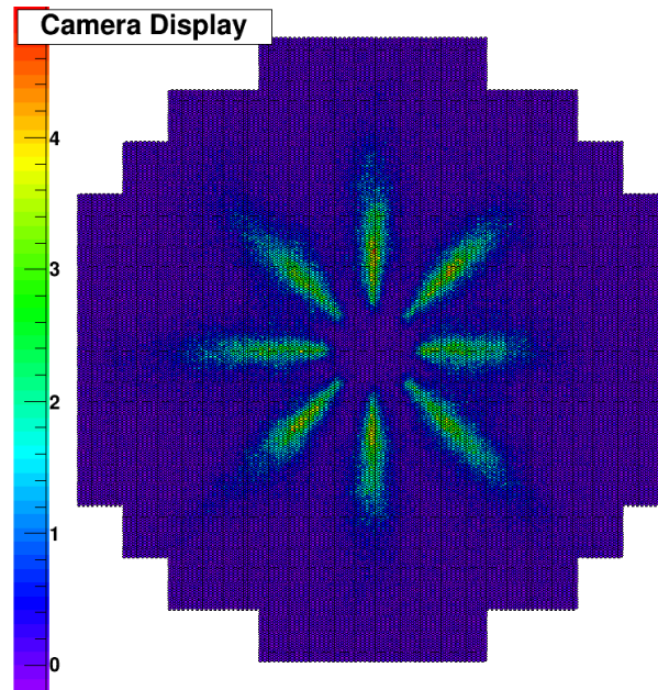
FIGURE 4.2 – Simulation de 400 photons \gamma à 25 GeV avec un angle zénithal nul, un angle azimutal provenant du Sud, en l'absence de champ magnétique pour une distance d'impact de 100 m. Les photons proviennent dans ce cas de 8 directions différentes sur le ciel.
