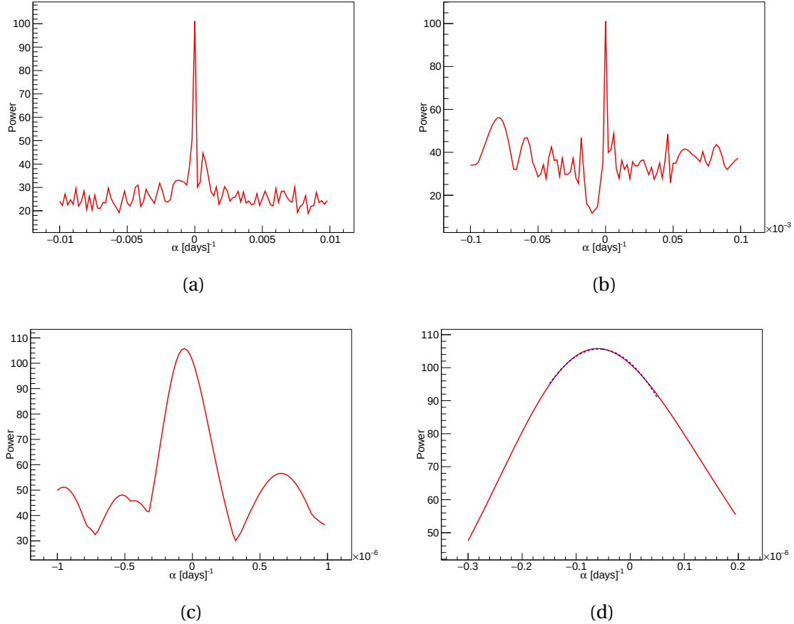
FIGURE 7.10 – Fonction résiduelle normalisée pour différents ordre de grandeur \alpha en jour -1 : (a) \alpha \in [-10^{-2}; 10^{-2}] ; (b) \alpha \in [-10^{-4}; 10^{-4}] ; (c) \alpha \in [-10^{-6}; 10^{-6}] et (d) \alpha \in [-3.0 \times 10^{-7}; 2.0 \times 10^{-7}] . La fonction résiduelle normalisée z est ajustée par une fonction parabolique et présente un maximum pour \alpha = -6.2 \times 10^{-8} jour -1 . Sur le graphe b, on voit apparaître également les harmoniques de ce paramètre \alpha .
