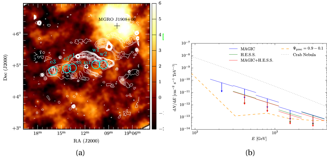
FIGURE 5.2 – (a) : Carte de signification, obtenue par H.E.S.S. pour un champ de vue centré sur la position de SS 433 à une énergie E \geq 287\text{GeV} . Les contours de radio GB6 à f = 4.85\text{ GHz} (en blanc, de Gregory et al. [41]) sont superposés. Les cercles cyan indiquent les positions des régions d'interaction e1, e2, e3 (à l'Est) et w1, w2 (à l'Ouest). La source lumineuse située au nord-ouest de SS 433 est MGRO J1908 + 06 [54].
