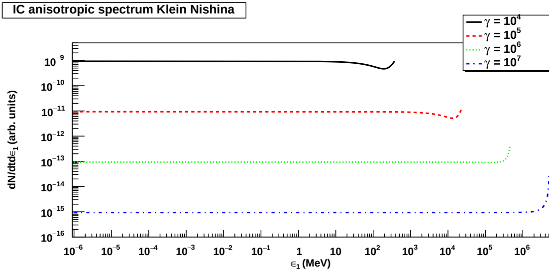
FIGURE 6.4 – Spectre en régime de Klein–Nishina \theta_0 = \pi , \epsilon_0 = 1 eV pour différentes valeurs de \gamma . Le spectre devient extrêmement asymétrique à haute énergie [6] [9]. Comparé à la figure 6.3, le spectre de la production des photons \gamma est dans ce cas limité en énergie.
