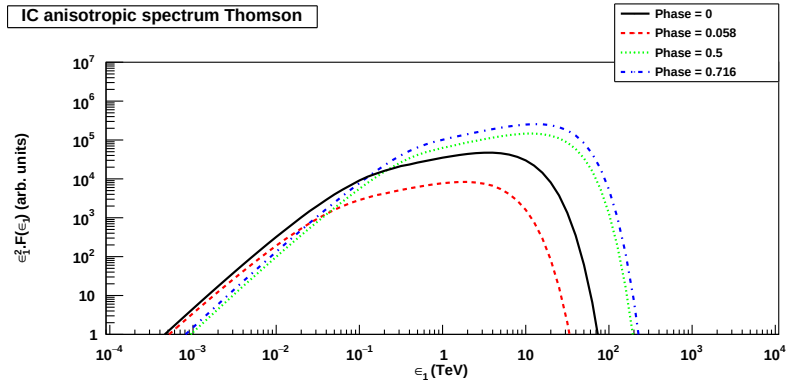
(b) Modèle de Thomson pour une inclinaison de 60^\circ
