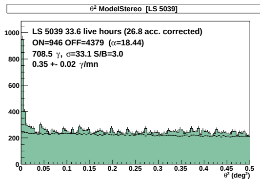
FIGURE 7.5 – Détermination du \theta^2 de la source pour une analyse H.E.S.S. phase II. Il est plus difficile de normaliser à \theta^2 = 0.5^{\circ 2} , il y a une contamination inévitable par HESS J1825–137.
