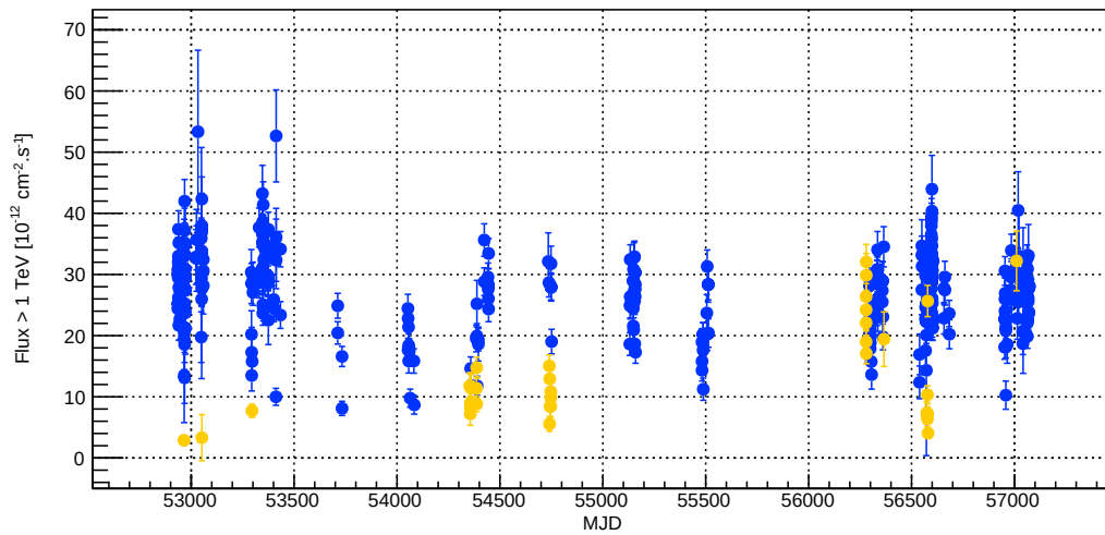
FIGURE 3.21 – Courbe de lumière de la nébuleuse du Crabe. Les observations pour lesquelles \text{TC} < 0.70 sont représentées en orange.
