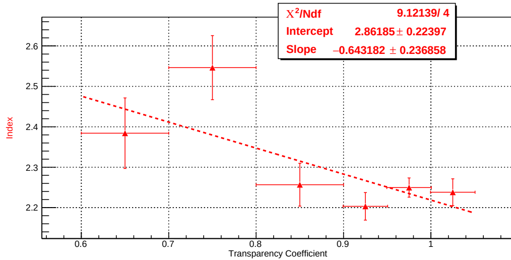
FIGURE A.10 – Influence de la transparence de l’atmosphère sur l’indice spectral mesuré système binaire LS 5039.
