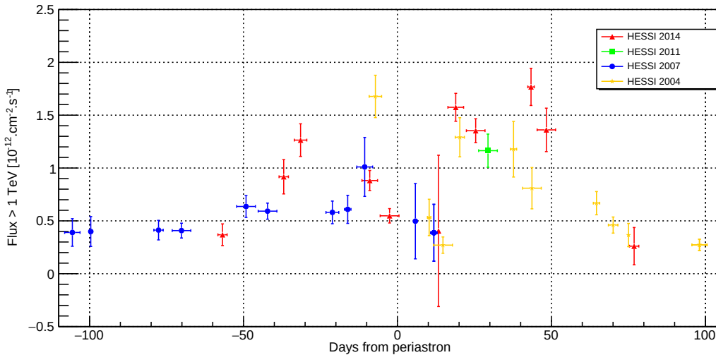
FIGURE 8.6 – Courbes de lumière repliées sur la phase avec un intervalle au niveau du temps d'une semaine pour les campagnes d'observations de 2004 (en jaune), 2007 (en bleu), 2011 (en vert) et 2014 (en rouge). Les points ont été extraits à partir d'une analyse de type HESS I. Les indices spectraux pour la détermination des valeurs points la courbe de lumière sont ceux de chaque campagne.
