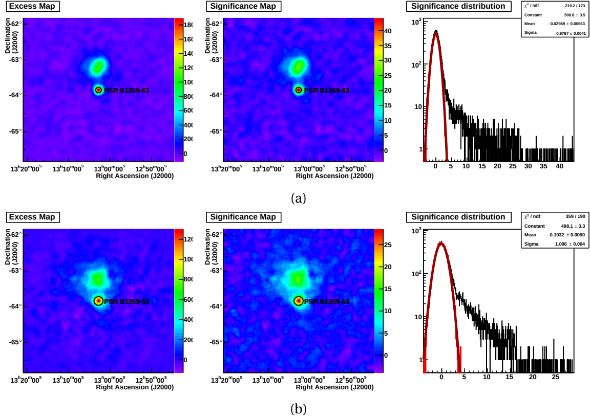
FIGURE 8.2 – Carte d'excès, de signification et de distribution du fond avec les analyses STEREO CT1-5 (a) et MONO (b).
