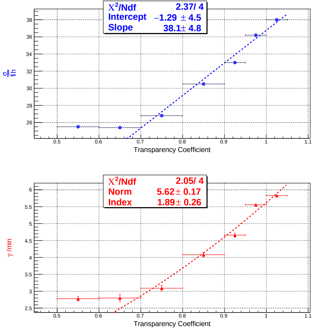
FIGURE 3.17 – Influence du coefficient de transparence sur la valeur de la signifi- cance de la nébuleuse du Crabe corrigée par le temps \frac{\sigma}{\sqrt{h}} (figure du haut) et sur le nombre de photons \gamma détectés par minute (figure du bas). Les courbes sont ajustées sur l'intervalle TC \in [0.60 ; 1.05] , un palier minimal apparaît en-dessous de ces valeurs. Les fonctions obtenues sont : \frac{\sigma}{\sqrt{h}} = a.TC + b avec b = 38.1 \pm 4.9 et a = -1.3 \pm 4.5 et \gamma / \text{min} = K.TC^\alpha avec K = 5.62 \pm 0.17 et \alpha = 1.89 \pm 0.26 . Un palier est observé pour un coefficient de transparence inférieur à 0.7.
