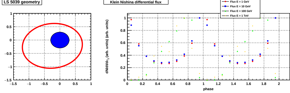
FIGURE 6.11 – Flux différentiel simulé à différentes énergies (1 GeV en rouge, 10 GeV en bleu, 100 GeV en vert et 1 TeV en jaune) pour différentes positions de l'objet compact dans le système binaire LS 5039 avec une orbite inclinée de 30^\circ par rapport à l'observateur
