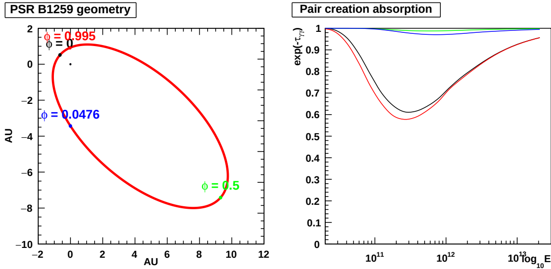
FIGURE 8.11 – Géométrie et absorption en fonction de l'énergie pour différentes phases pour le système binaire PSR B1259-63. Le phénomène d'absorption est non négligeable lorsque l'objet compact se trouve au niveau de la conjonction supérieure pour une énergie se situant sur un intervalle 100 GeV - 1 TeV. Cette courbe d'absorption correspond à une interaction entre les photons de l'étoile Be et les photons \gamma produits.
