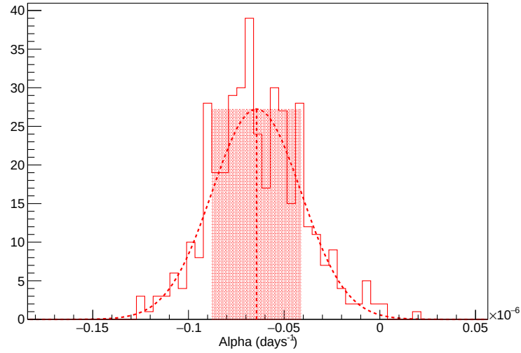
FIGURE 7.11 – Détermination de la précision du paramètre \alpha à partir de 400 courbes de lumière générées aléatoirement à 1\sigma . L'histogramme est ajusté par une gaussienne ce qui permet d'obtenir la précision du paramètre \alpha .
