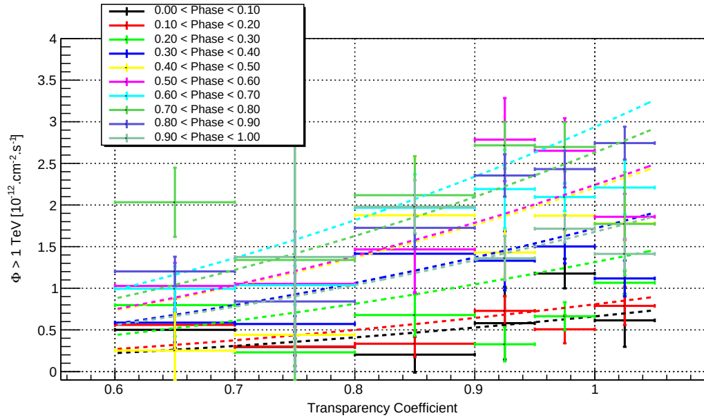
FIGURE A.13 – Influence du coefficient de transparence sur le flux intégré mesurée au-dessus de 1 TeV pour chaque phase de LS 5039.
