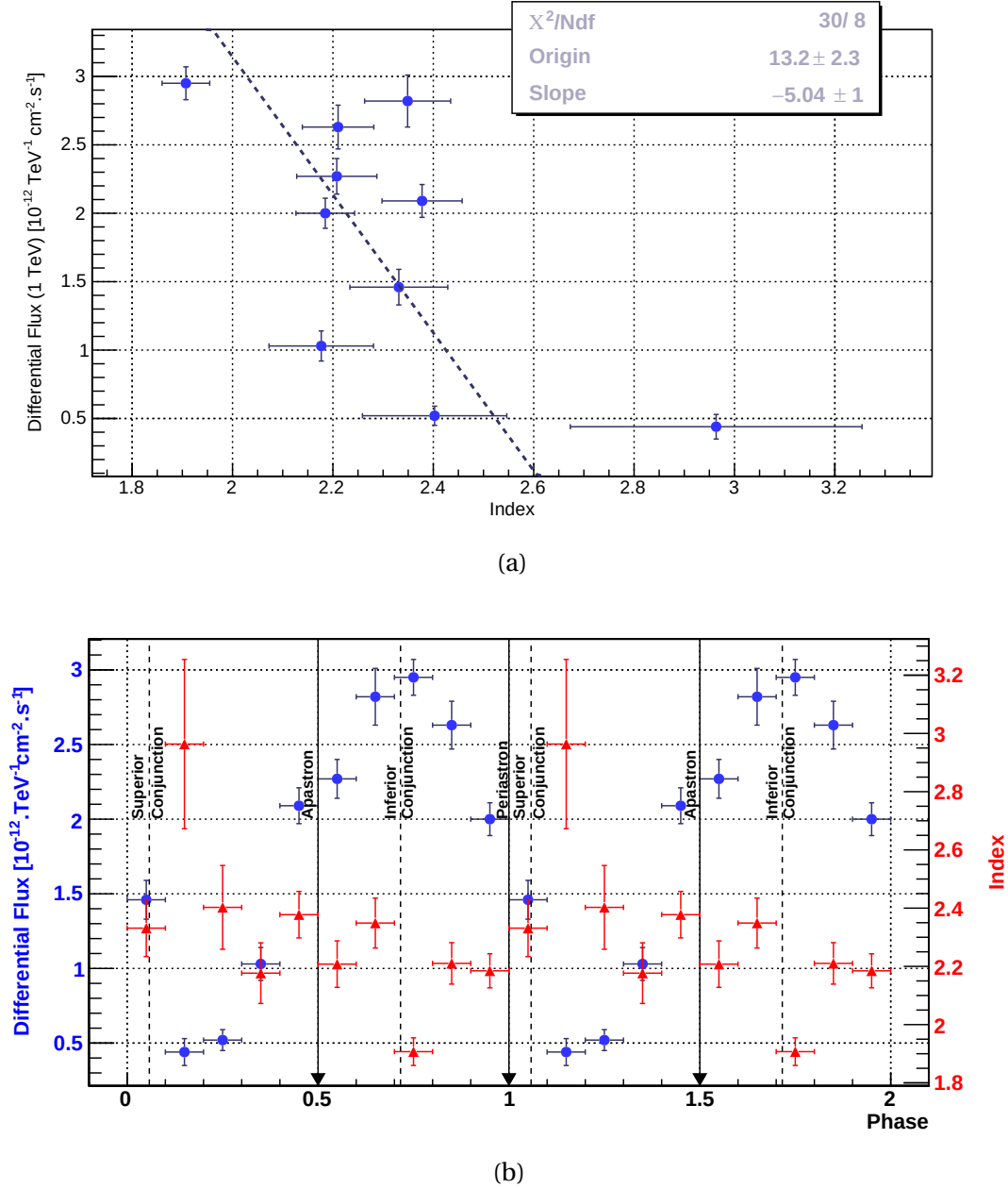
FIGURE 7.15 – Flux différentiel et indice spectral pour chaque phase de LS 5039 avec une analyse H.E.S.S. phase I. Sur le graphe (a) ces deux grandeurs sont représentées et ajustées par une droite affine. La pente négative de la droite indique un comportement d'anticorrélation entre des deux grandeurs. Sur le graphe (b), on a représenté les mêmes valeurs (flux différentiel à 1 TeV en bleu et indice spectral en rouge) pour deux orbites de LS 5039. Les positions particulières de l'objet compact sur son orbite sont indiquées par des traits verticaux en pointillés ou des flèches.
