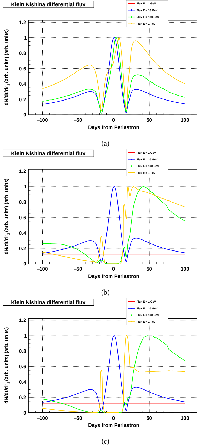
FIGURE 8.14 – Flux différentiel simulé par une émission inverse anisotrope Compton Klein–Nishina en tenant compte du disque circumstellaire de l’étoile compagnon et des effets de créations de paires pour différentes températures du disque circumstellaire : 6300 K (a) 18500 K et (b) 22500 K (c).
