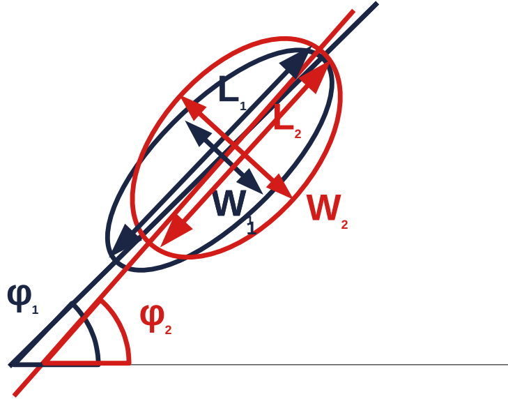
FIGURE 4.5 – Définition des paramètres de correction de la rotation de l'image : \Delta\phi , \Delta L et \Delta W .
