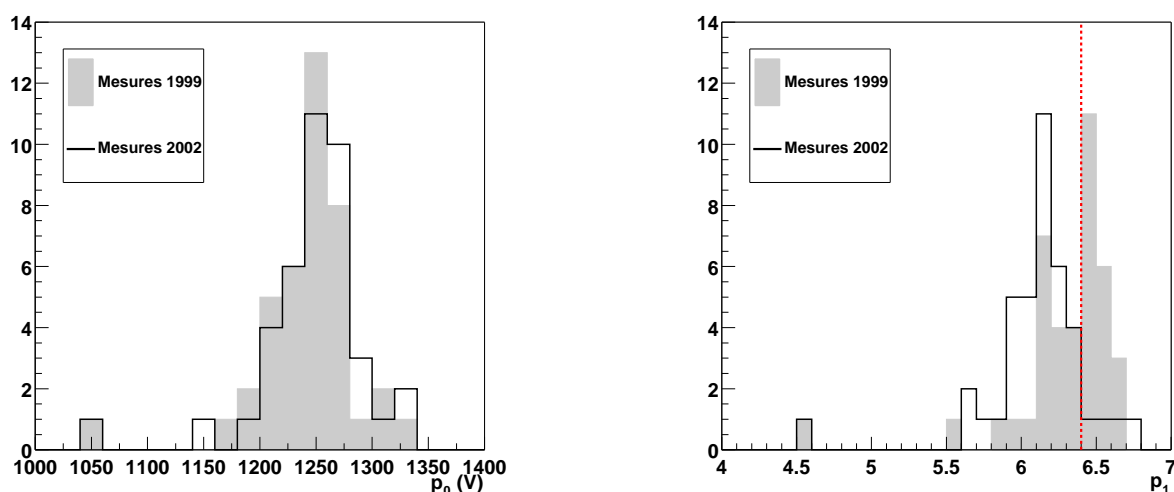
FIG. 4.9 . Vieillesse des photomultiplicateurs. Comparaison des paramètres p_0 (à gauche) et p_1 (à droite) tels que mesurés en 1999 et en 2002. La ligne verticale indique la valeur attendue de p_1 pour un photomultiplicateur neuf.
