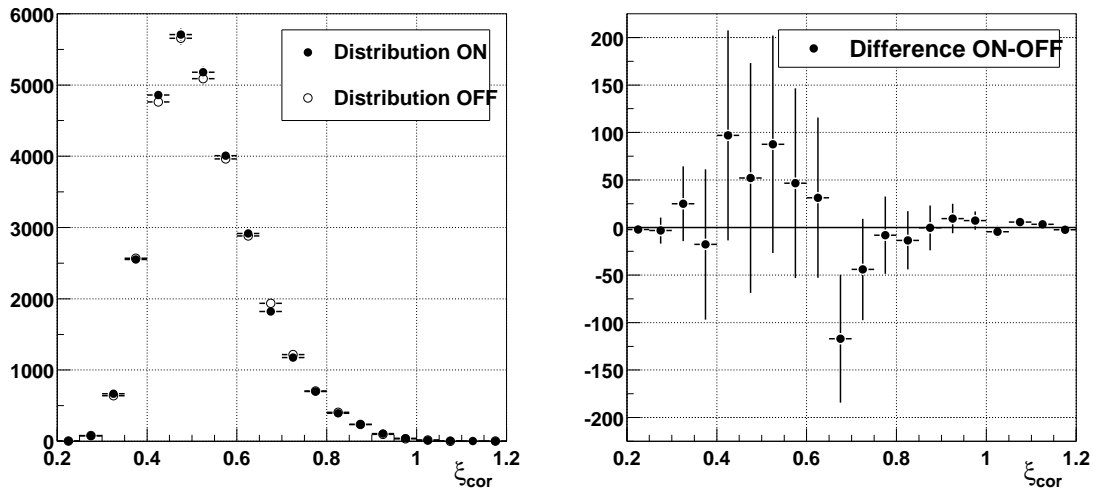
FIG. 10.11 . Distributions de \xi_{\text{cor}} pour les données IES1426+428 ( N_V=0 ). À gauche : distributions ON et OFF de la variable \xi_{\text{cor}} pour les données IES1426+428 après coupure sur N_V ( N_V = 0 ). À droite, différence ON-OFF de ces mêmes distributions.
