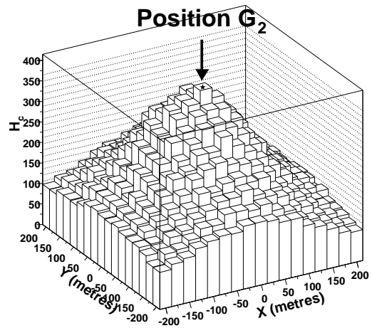
FIG. 8.6 . Recherche du point d'impact de la gerbe (2). À gauche : Deuxième étape de la recherche, sur une grille fine. En encart sont représentés les profils des distributions H_c suivant X et Y, ainsi que l'ajustement par une lorentzienne permettant d'obtenir la position du point d'impact. À droite : Distribution des valeurs H_c pour chaque position de la grille est donnée.
