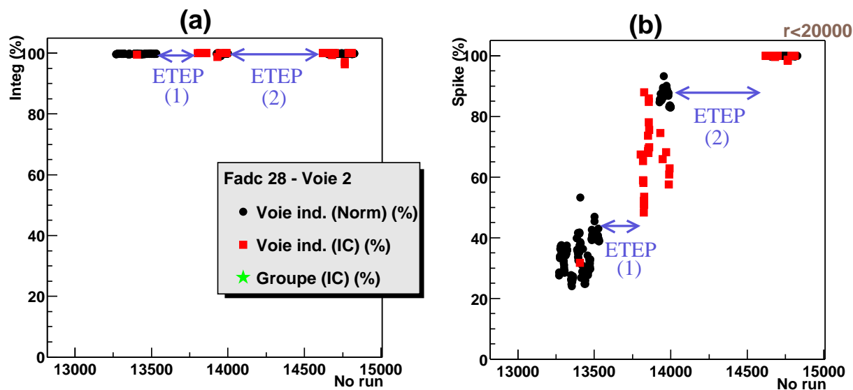
FIG. 5.7 . Évolution des estimateurs de qualité I et S dans le temps. L'indication « ETEP » se rapporte au passage de la carte dans les ateliers d'EETEP.
