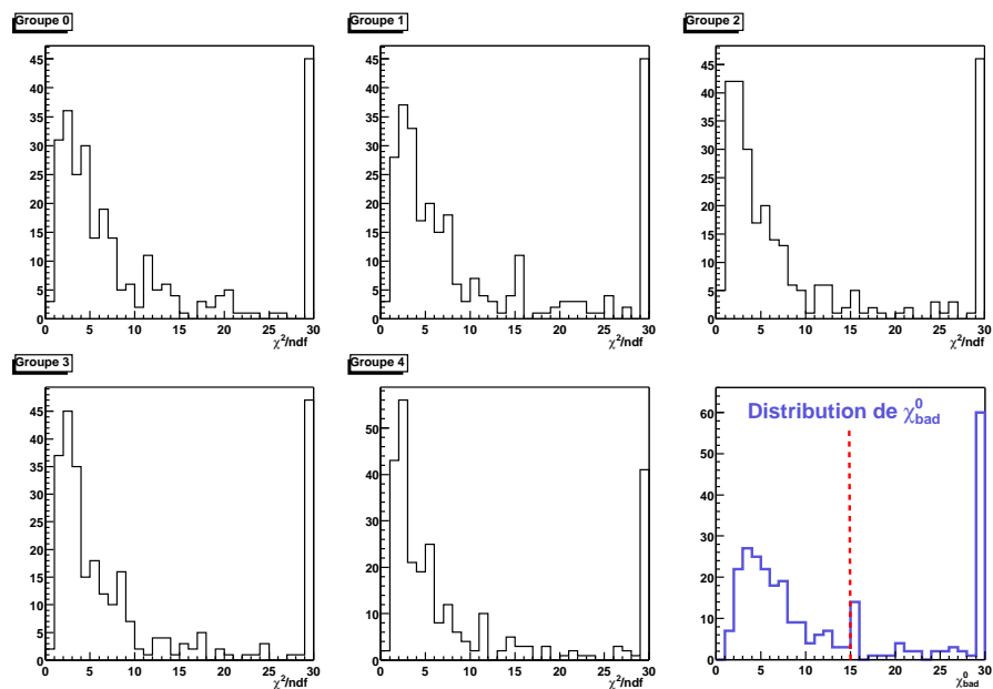
FIG. 6.6 . Distribution des valeurs des \chi^2/\text{ndf} pour chaque groupe de déclenchement. La dernière distribution est celle de la variable \chi_{bad}^0 , la ligne pointillée indique la coupure appliquée dans la suite.
