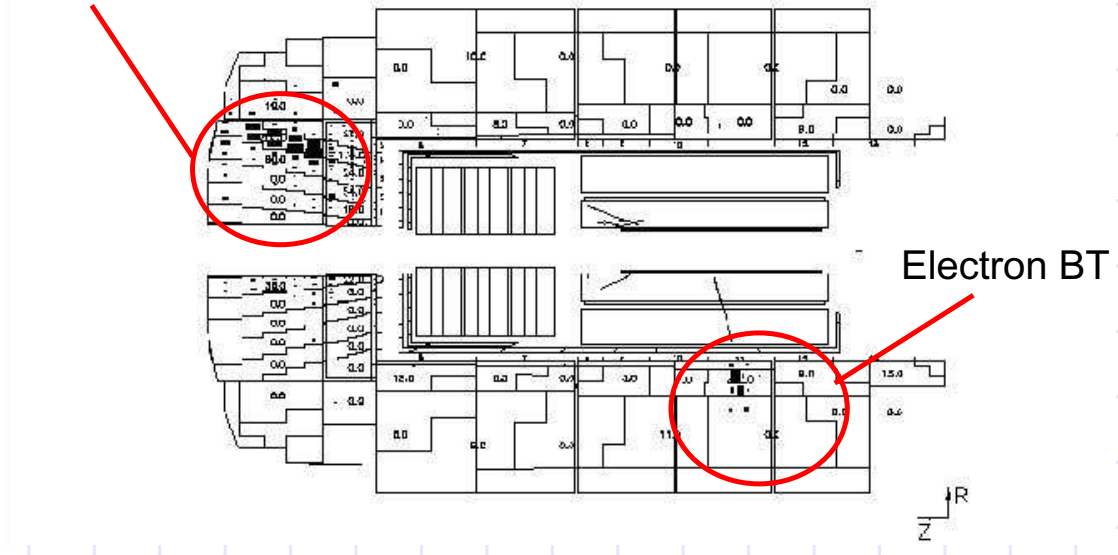
Figure 5.3: Exemple d'un événement où S67 a été déclenché par l'électron diffusé et le HFS (source communication interne de A. Nikifrov).
