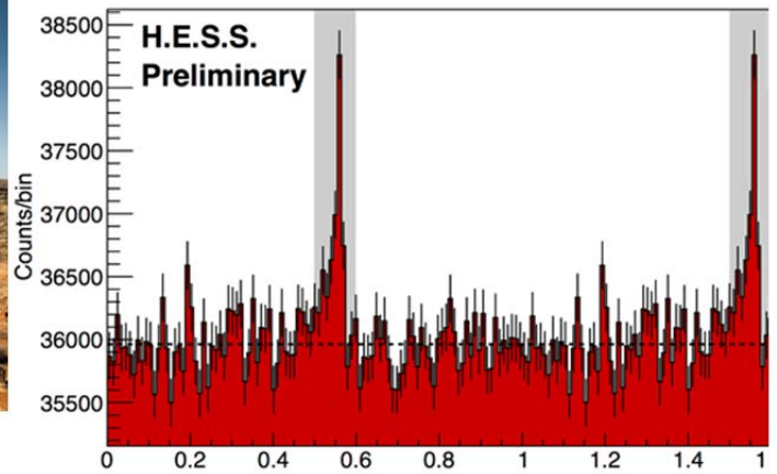
Émission périodique de rayons gamma en provenance du pulsar de Vela, telle que mesurée par l'expérience H.E.S.S. Une période correspond à 89 millisecondes. En abscisse, sont représentées les phases de la période du pulsar. © collaboration H.E.S.S.
